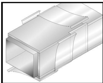
Rys.1 Powłoka Aluminio 374 docinana na wymiar z zalecaną zakładką 75mm.
