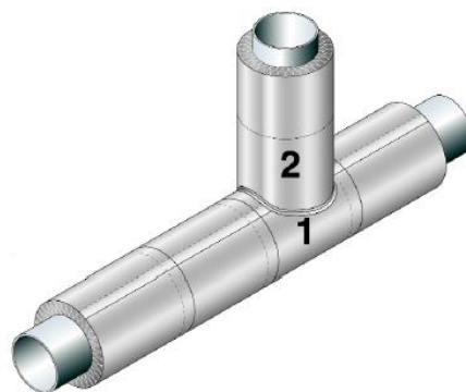
Rys.8 Izolacja trójników.
